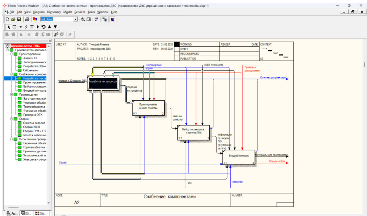
Рисунок 4 – декомпозиция процесса «Снабжение компонентами»
