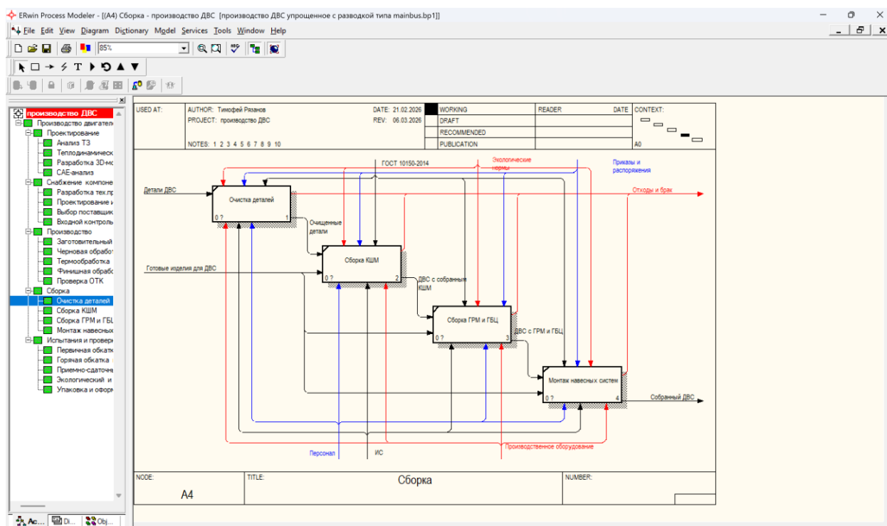
Рисунок 6 – декомпозиция процесса «Сборка»
