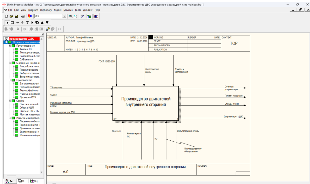
Рисунок 1 – контекстный уровень IDEF0
